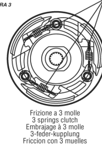
MOLLE DA SOSTITUIRE - SPRINGS TO BE REPLACED RESSORTS À REMPLACER - ZU ERSETZENDE FEDER MUELLES PARA SUSTITUCIÓN
