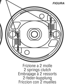
MOLLE DA SOSTITUIRE - SPRINGS TO BE REPLACED RESSORTS À REMPLACER - ZU ERSETZENDE FEDER MUELLES PARA SUSTITUCIÓN
