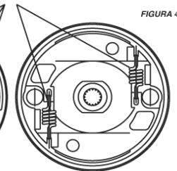
MOLLE DA SOSTITUIRE - SPRINGS TO BE REPLACED RESSORTS À REMPLACER - ZU ERSETZENDE FEDER MUELLES PARA SUSTITUCIÓN
