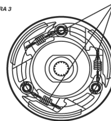
MOLLE DA SOSTITUIRE - SPRINGS TO BE REPLACED RESSORTS À REMPLACER - ZU ERSETZENDE FEDER MUELLES PARA SUSTITUCIÓN
